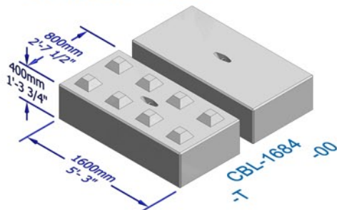
Bloc Régulier Mi-Hauteur
