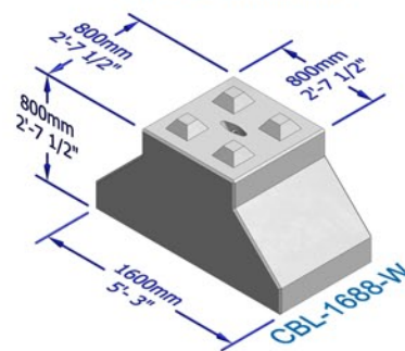
Bloc de Fondation
